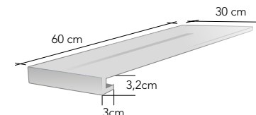
GRADINO ANGOLARE COSTA RETTA (sx/dx) 30x60x3,2x3 - 12"x24"x1.2"x1"
