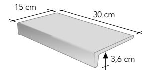
elemento continuativo ELLE 15x30x3,6 - 6"x12"x1.4"
