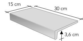
elemento continuativo ELLE 15x30x3,6 - 6"x12"x1.4"
